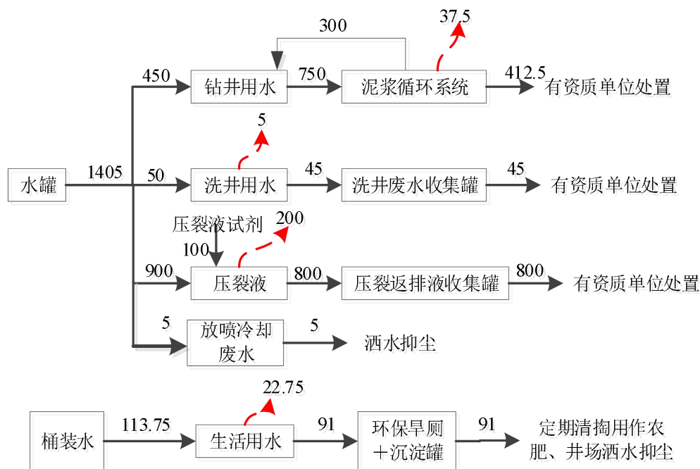
图 2-2 项目水平衡图 (单位: m³)
