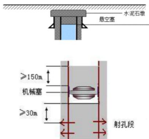
图 2-6 永久封井示意图
