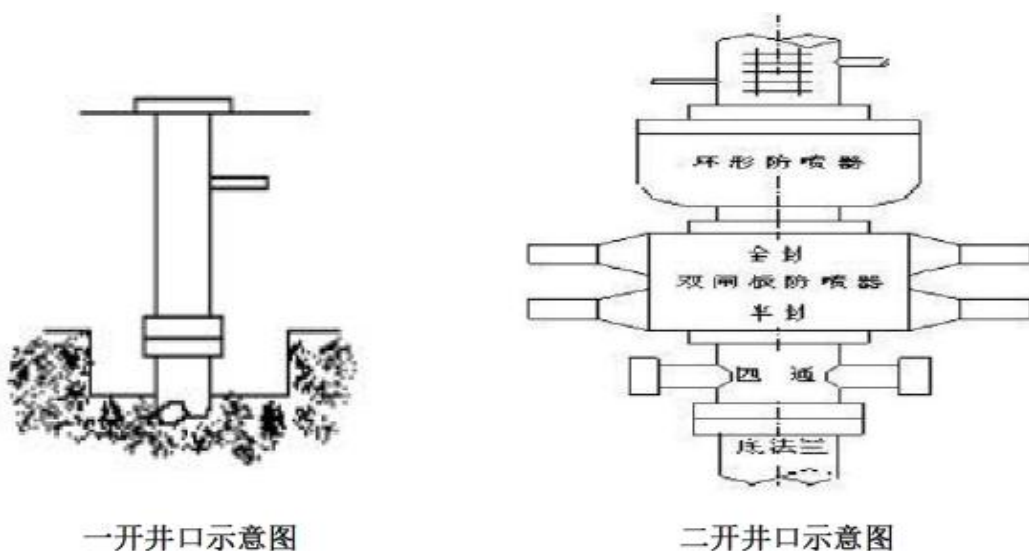
图 2-4 一开、二开井口示意图
