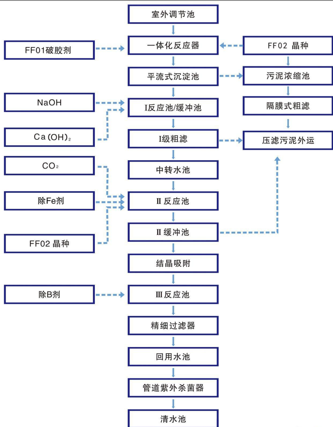
图 5-4 水处理工艺流程图
