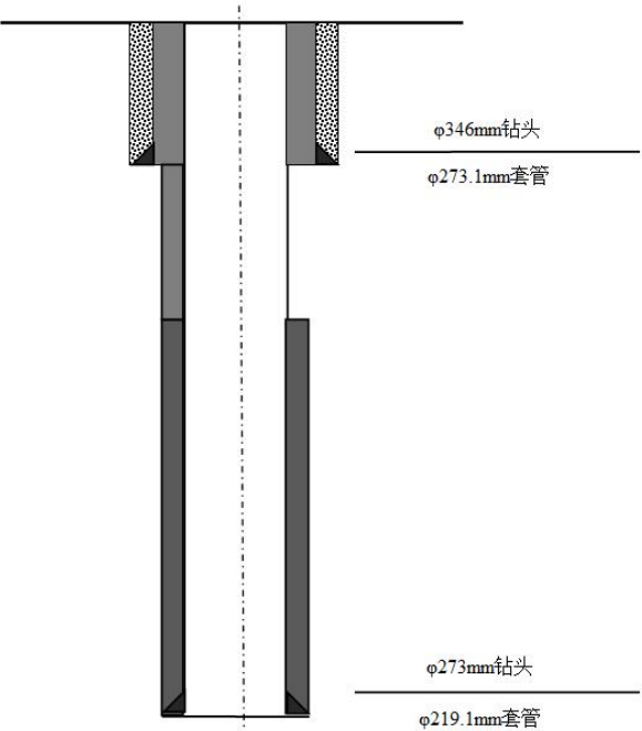
图 2-1 井身结构图
