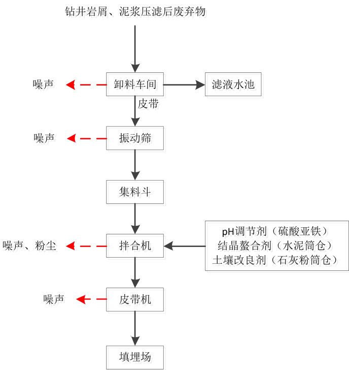
图 5-6 陕西德禾鑫盛环保科技有限公司工艺流程图
