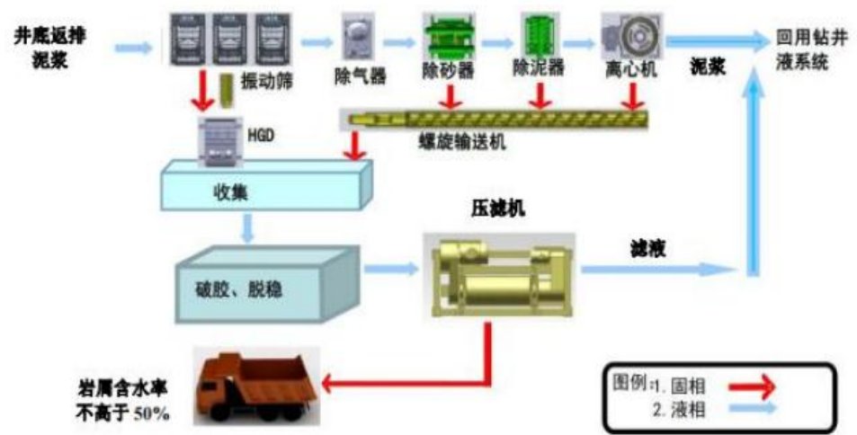
图 2-7 泥浆循环系统工艺流程简图
