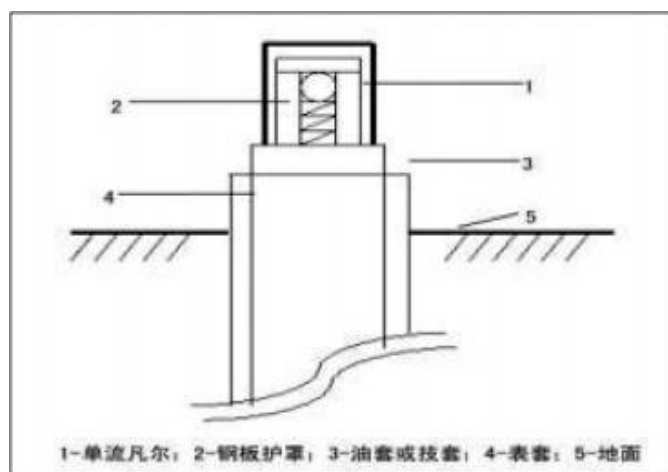
图 2-5 临时封井示意图
