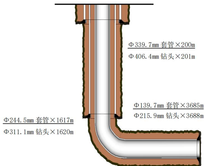
图2-2 佳页1H井身结构示意图
