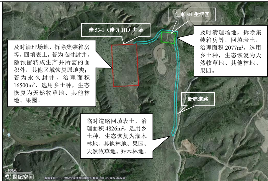
图5-2 佳53-1（佳页1H）井场生态恢复措施示意图
