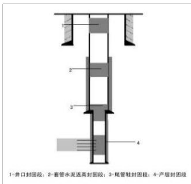
图2-4 永久封井剖面示意图
