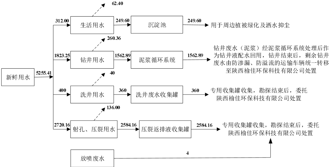
图2-5 项目水平衡图（单位：m³/施工期）
