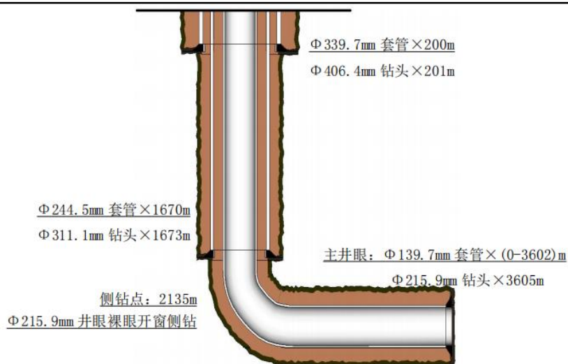
图2-1 佳南5H井身结构示意图
