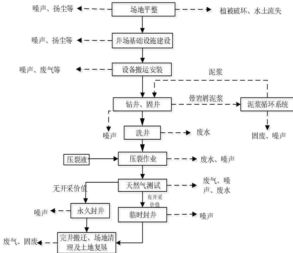
图2-7 项目主要工艺流程及产污环节
