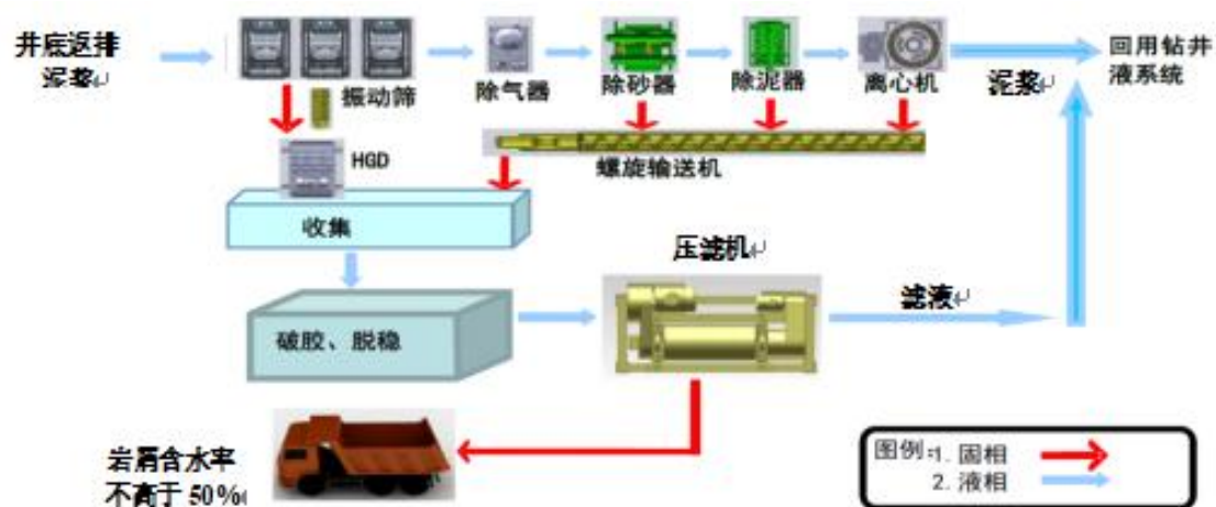
图2-6 泥浆循环系统工艺流程简图
