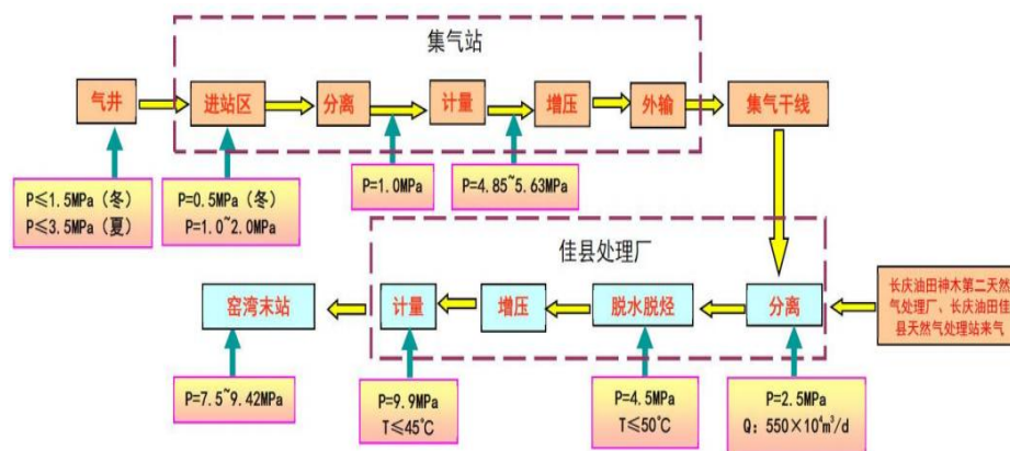
图 2-4 产能项目总体工艺流程图
