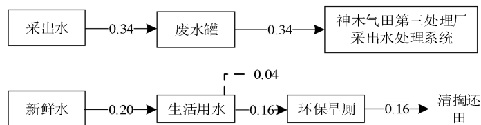
图 2-1 项目水平衡图 m³/d
