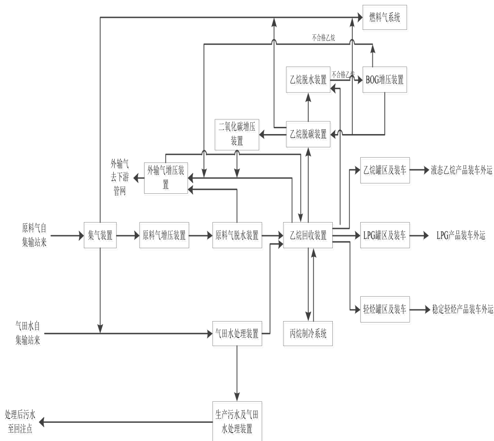
图 2-5 天然气处理厂总工艺流程图
