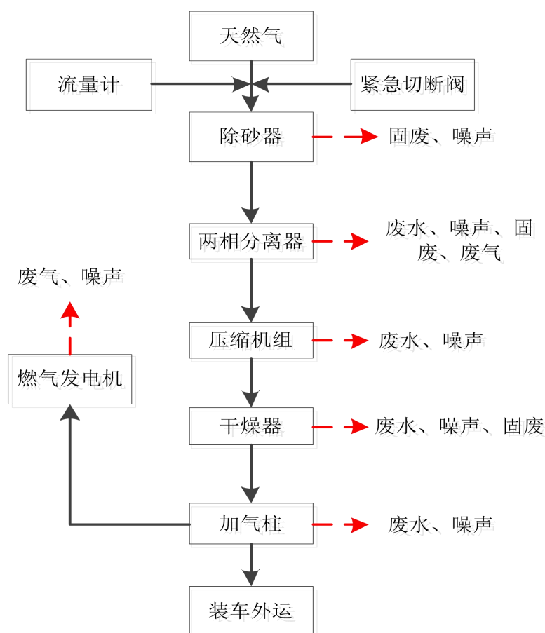
图 2-3 营运期工艺流程与产污环节图
