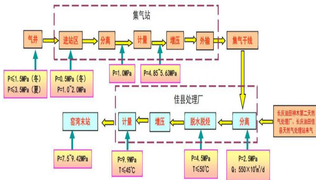
图 2-4 产能项目总体工艺流程图
