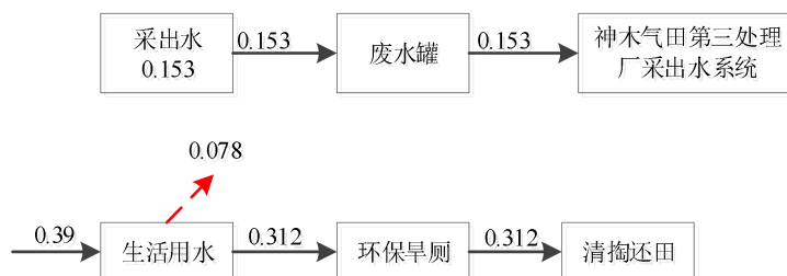
图 2-1 项目水平衡图 \text{m}^3/\text{d}
