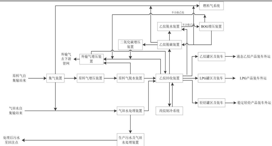
图 2-5 天然气处理厂总工艺流程图
