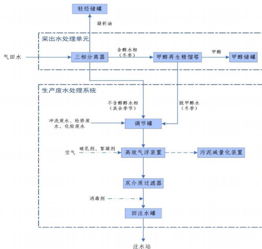
图 2-6 污水处理工艺流程图
