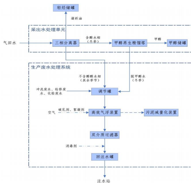
图 2-6 污水处理工艺流程图
