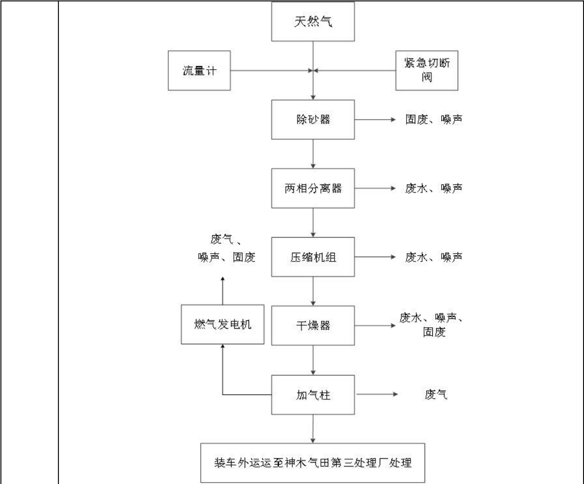
图 2-3 运营期工艺流程与产污环节图
