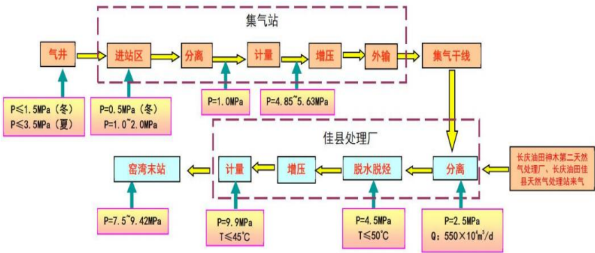
图 2-4 产能项目总体工艺流程图
