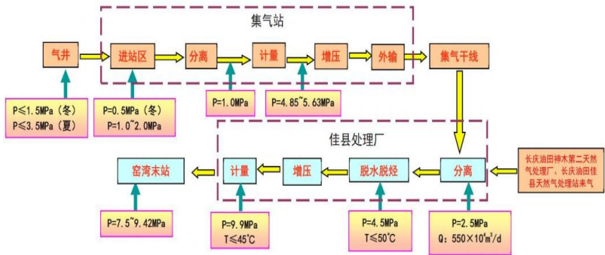
图 2-4 产能项目总体工艺流程图
