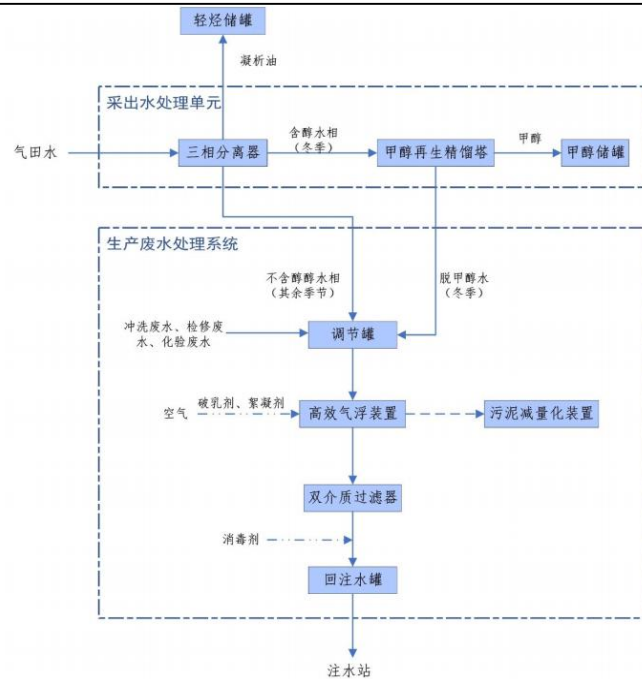
图 2-6 污水处理工艺流程图
