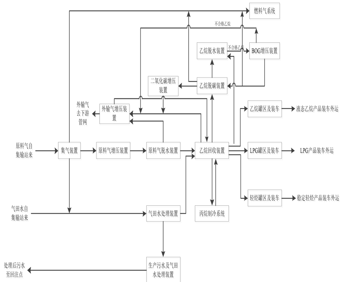
图 2-5 天然气处理厂总工艺流程图
