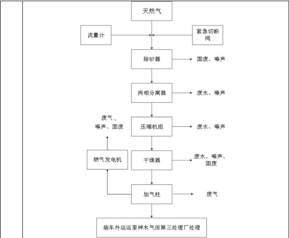
图 2-3 营运期工艺流程与产污环节图
