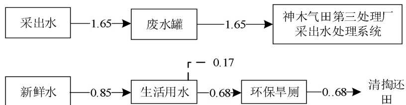
图 2-1 项目水平衡图 m³/d
