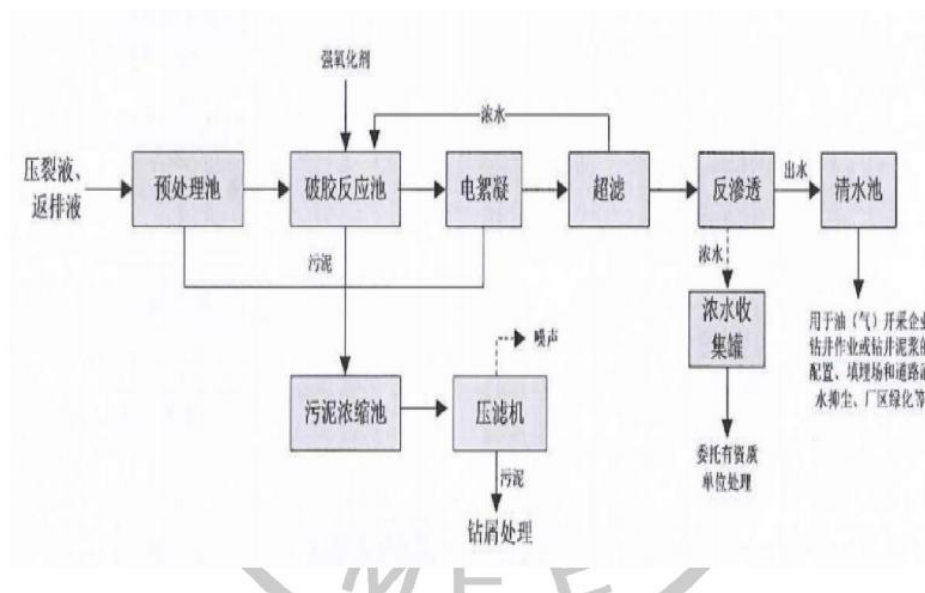
图 5-2 水处理工艺流程图
