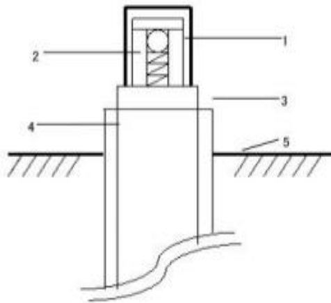
图 2-5 临时封井示意图
