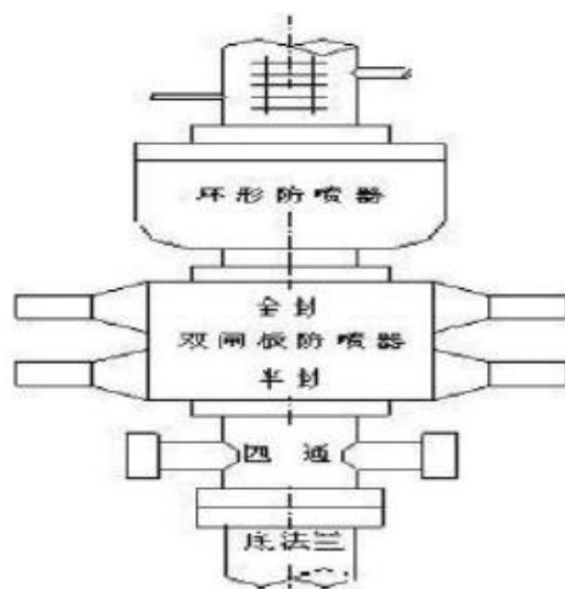
二开井口示意图
