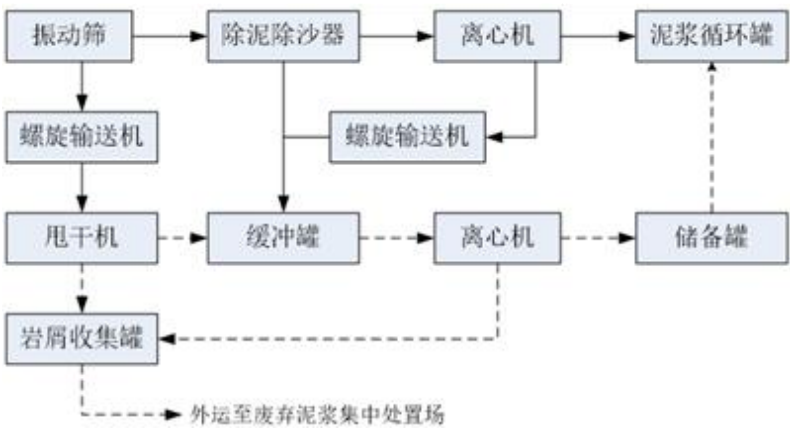
图 5-3 泥浆循环利用工艺流程图
