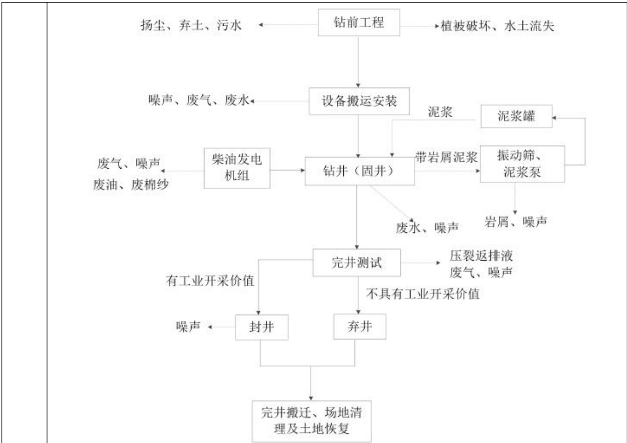
图 2-3 项目主要工艺流程及产污环节图
