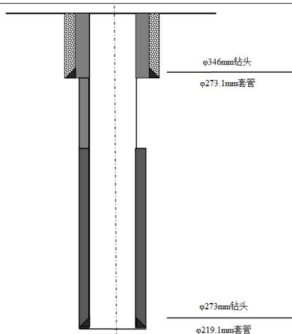
图 2-1 井身结构图
