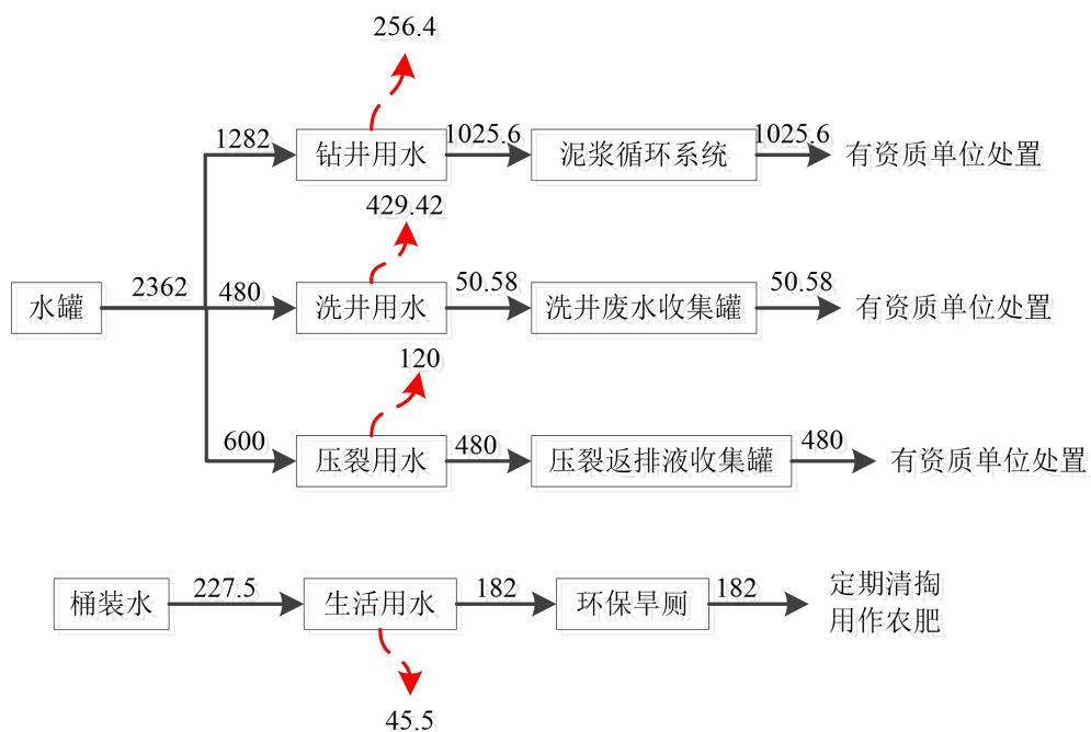
图 2-2 项目水平衡图（单位：m³/井）
