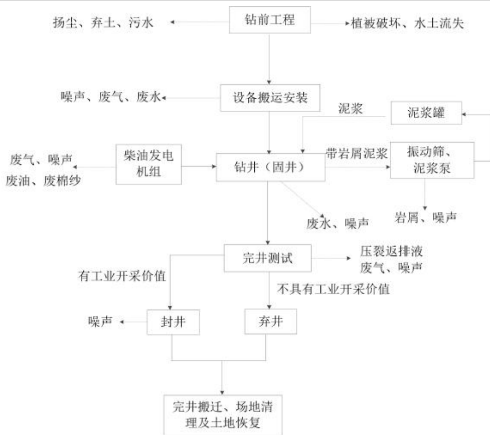
图 2-3 项目主要工艺流程及产污环节图
