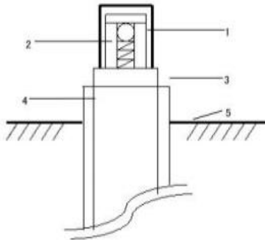
图 2-5 临时封井示意图
