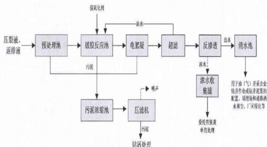
图 5-2 水处理工艺流程图
