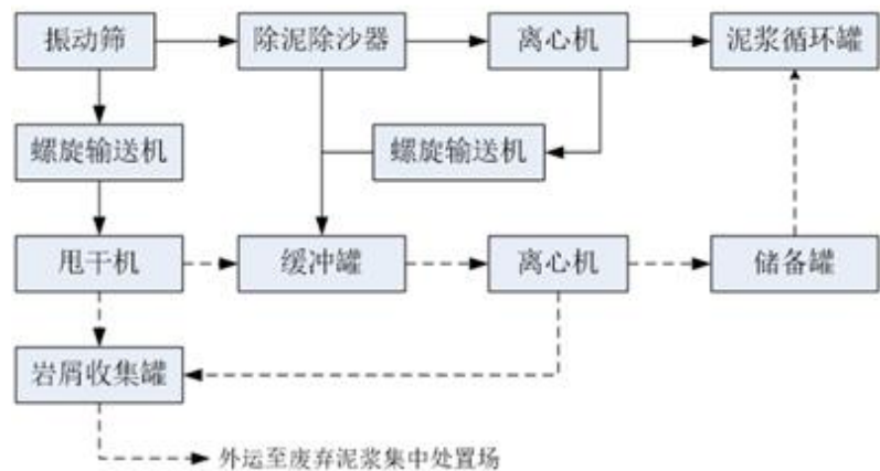
图 5-3 泥浆循环利用工艺流程图
