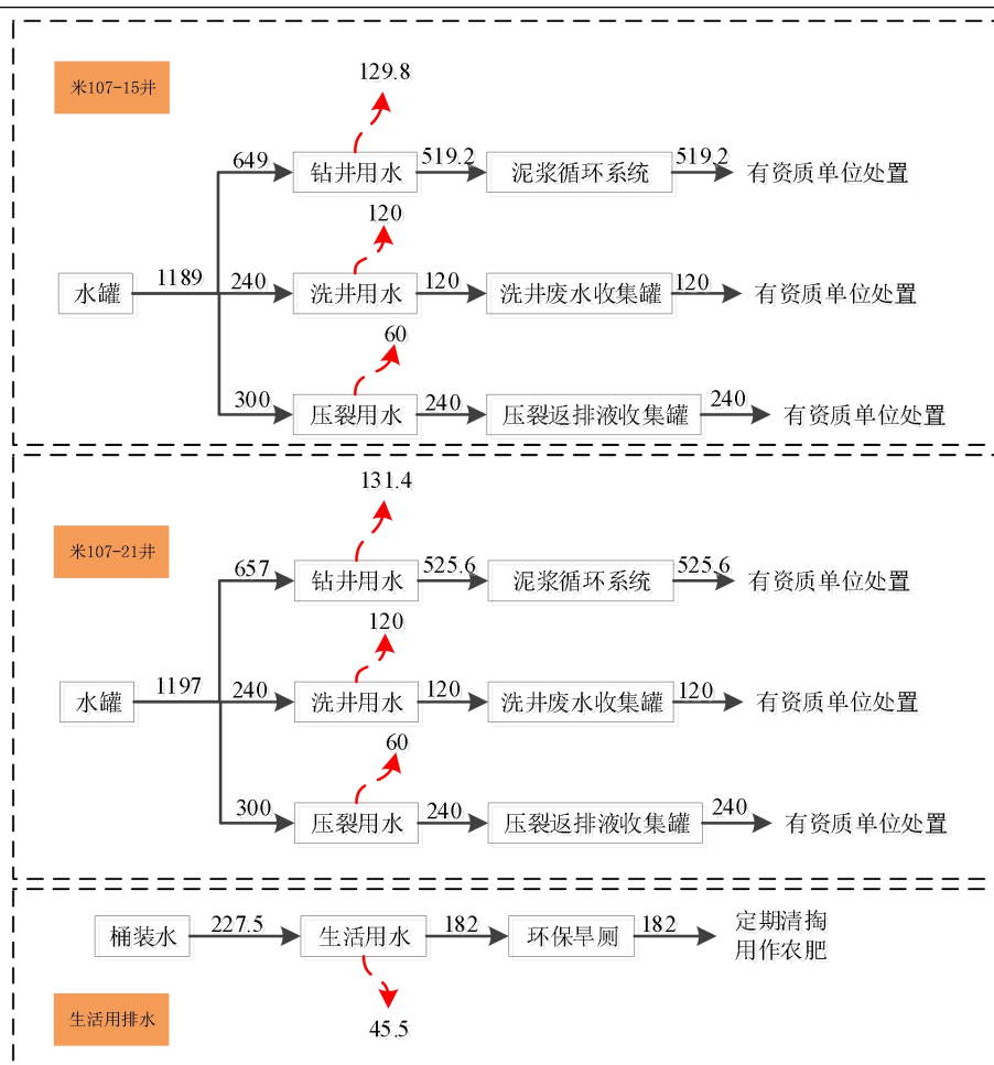
图 2-2 项目水平衡图（单位：m³/井）
